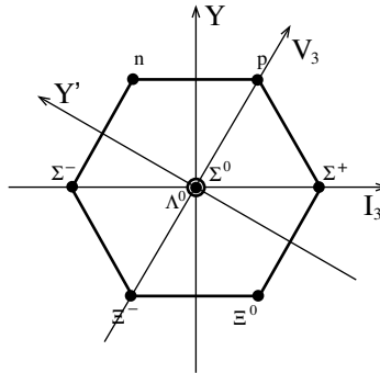
Fig. 8.10. I -spin and V -spin for the baryon octet.
